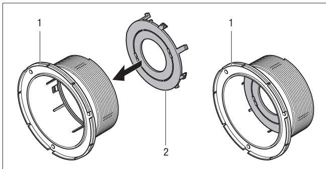
1 Anschlussstutzen, Ausströmseite 2 Luftregulierelement
