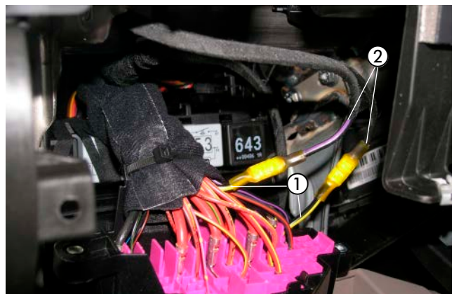
Abb. 46 ① Kabel 4 mm 2 sw/ge (Sicherung F40) ② Kabel 4 mm 2 sw und 4 mm 2 sw/vi einbinden
